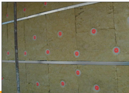
Die Beispielapplikation des ISOVER Maxil
