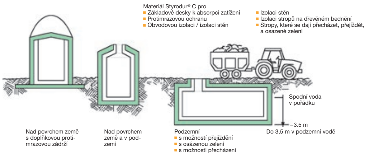
Obr. 3: Tepelná izolace s materiálem Styrodur® C u různých zařízení pro kvašení.
