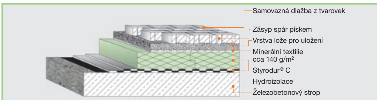
Obr. 4: Konstrukce střechy pro parkoviště se samovaznou dlažbou z tvarovek uloženou na vrstvu lože.
