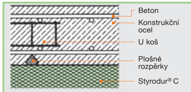
Obr. 19: Pochůzná plošná rozpěrka z vláknitého betonu pro spodní výztuž a opěrný koš z ocelového pleťo pro horní výztuž podlahové desky.
