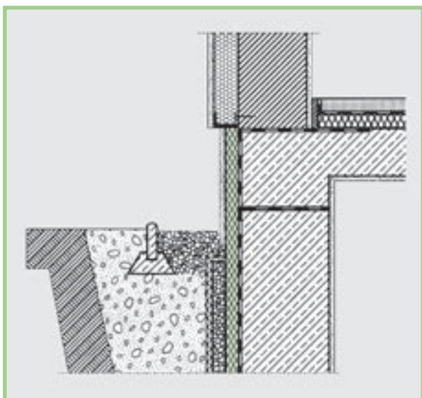
Obr. 12: Oblast soklu, izolace suterénu se sduženým tepelně izolačním systémem na vnější straně.
