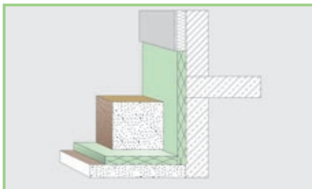
Obr. 28: Ochrana proti mrazu se klade do zeminy pod mrazovou hranici (max. hloubku promrzání).
