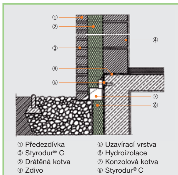
Obr. 31: Napojení izolace suteréru na zdivo s tepelnou izolací uvnitřskonzolovou kotvou.
