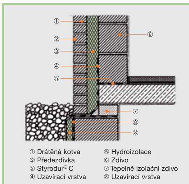
Obr. 30: Napojení izolace suteréru na zdivo s tepelnou izolací uvnitř.
