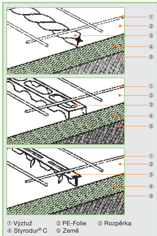
Obr. 20: Pochůzná plastové rozpěrky pro vodorovnou výztuž. Výškou profilu je dána výška překrytí betonu.
