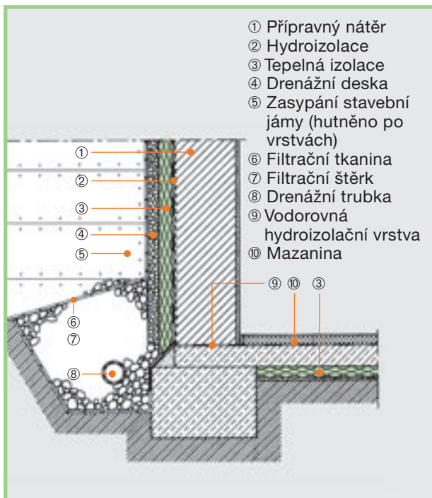
Obr. 24: Složení izolace suteréru kombinované s odvodněním.
