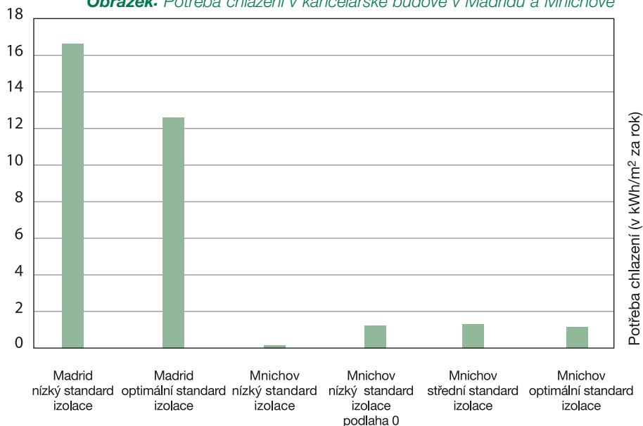
Obrázek: Potřeba chlazení v kancelářské budově v Madridu a Mnichově
